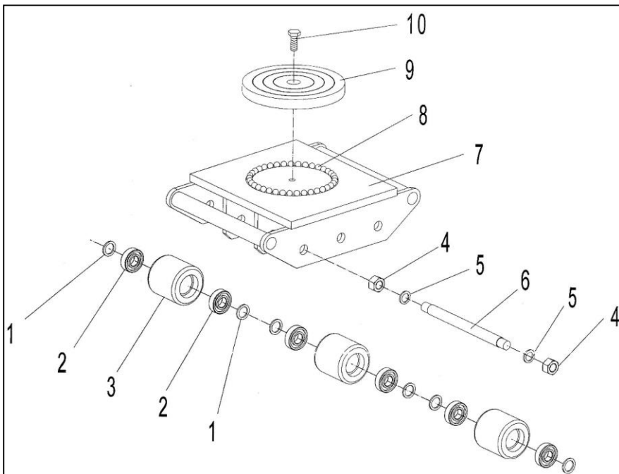
Схема 3. Платформа такелажная CRA-9.
